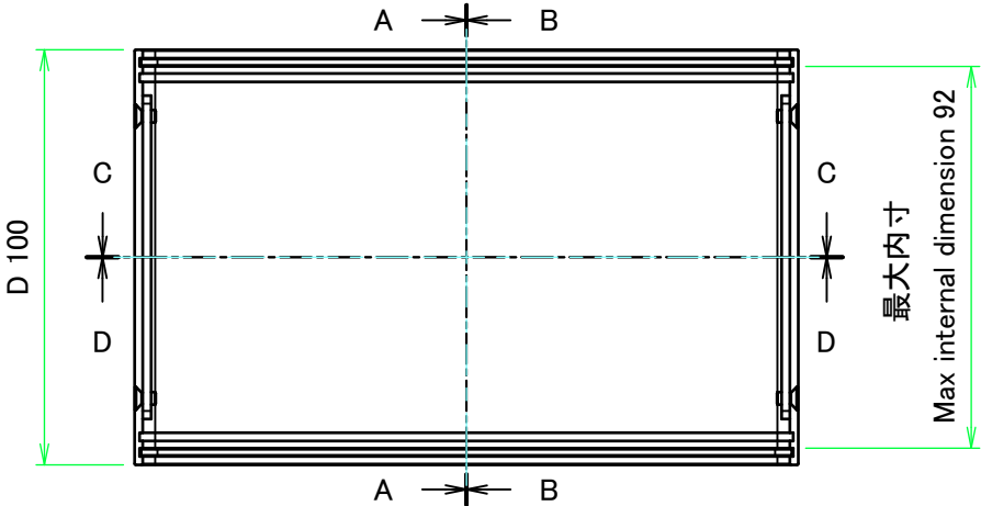
下カバー (内視) Bottom cover (Internal view)
