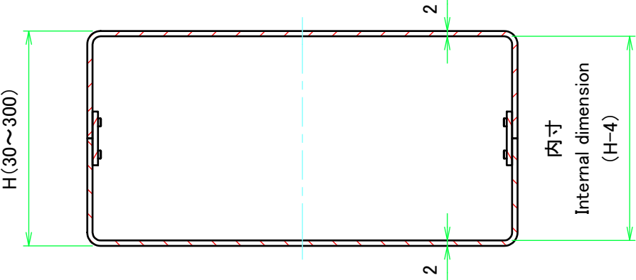
D-D ( 1 : 2 )
