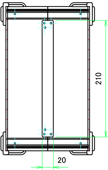
A-A ( 1 : 4 )
