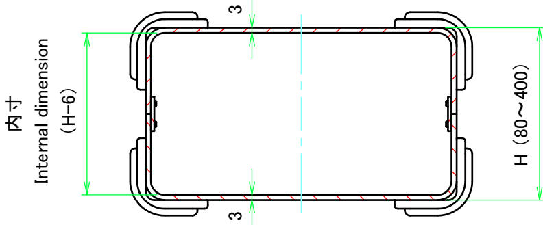
D-D (1:3)
