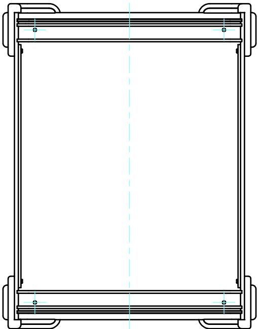
上カバー(内視) Top cover (Internal View)
