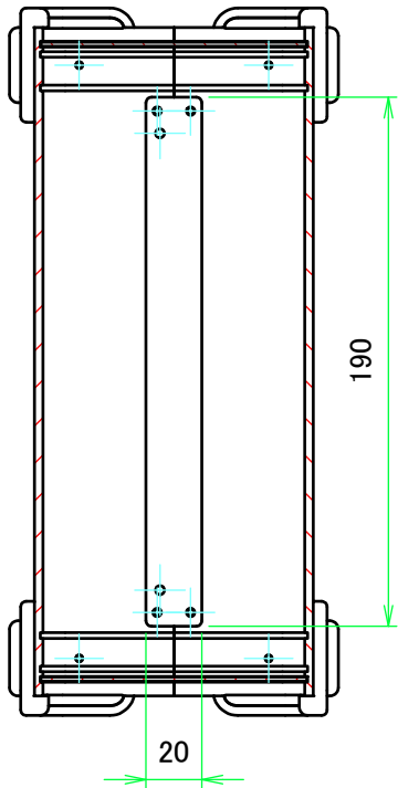
A-A (1:3)
