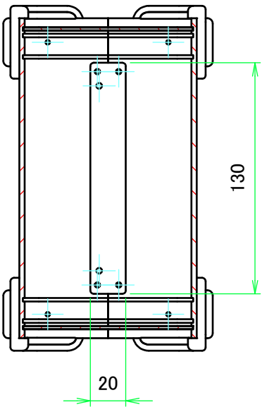
A-A (1:3)
