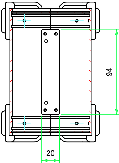
A-A ( 1 : 2.5 )
