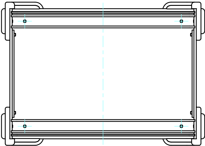
上カバー(内視) Top cover (Internal View)
