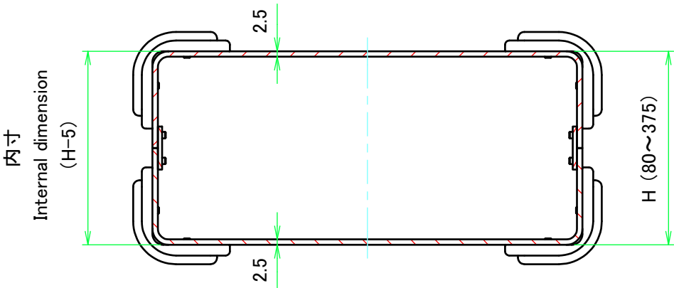
D-D ( 1 : 2.5 )
