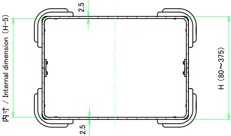
D-D ( 1 : 2.5 )
