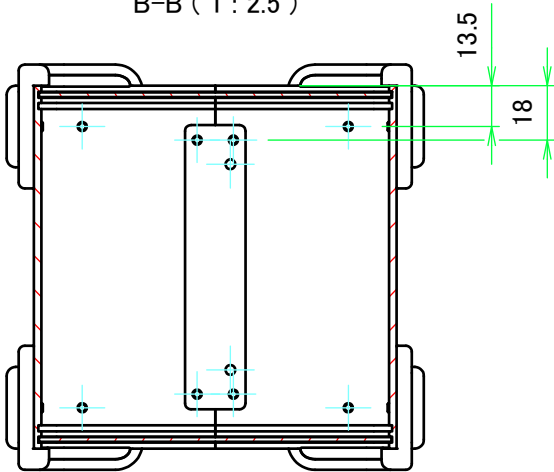
B-B ( 1 : 2.5 )
