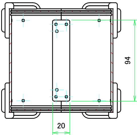
A-A ( 1 : 2.5 )
