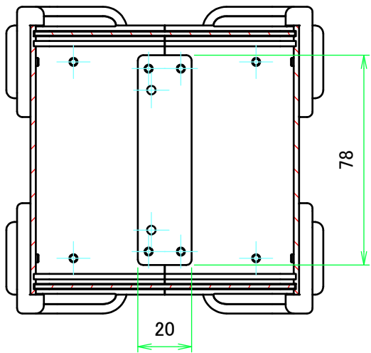
A-A ( 1 : 2 )
