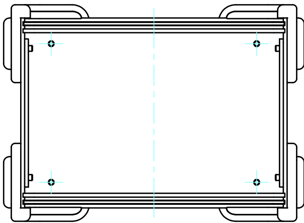
上カバー(内視) Top cover (Internal View)
