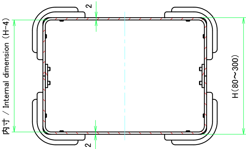
D-D ( 1 : 2 )
