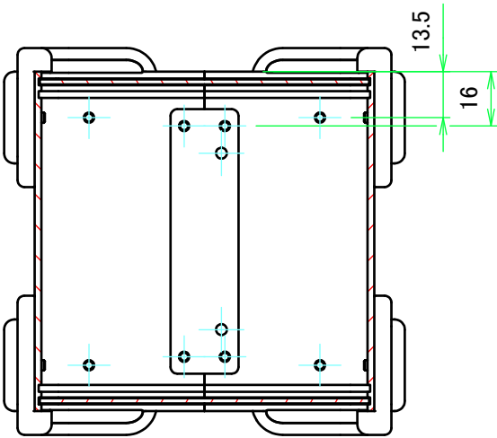
B-B ( 1 : 2 )
