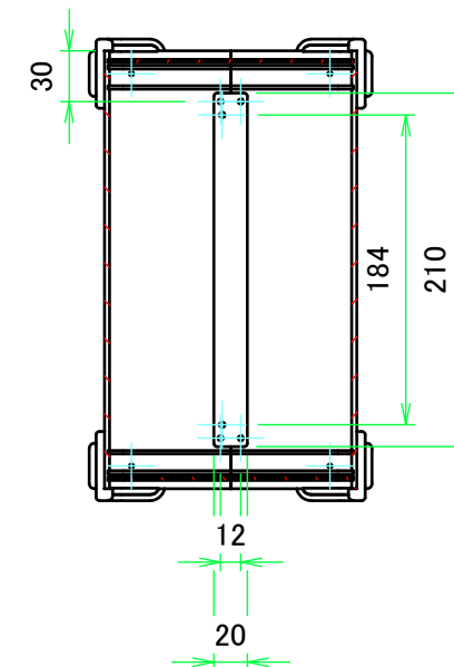
A-A ( 1 : 5 )
