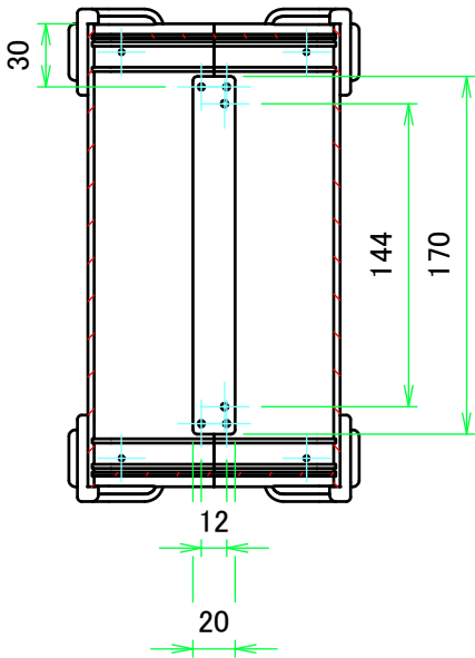
A-A ( 1 : 4 )
