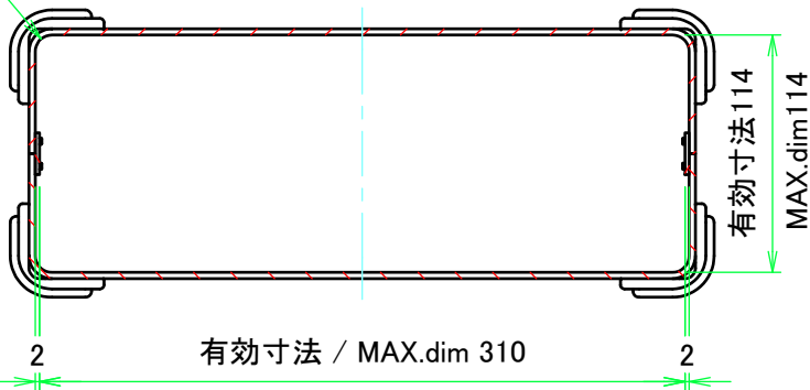
D-D ( 1 : 4 )
