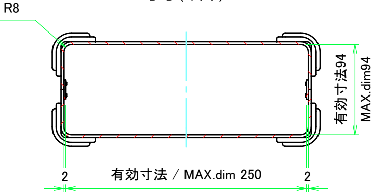
D-D ( 1 : 4 )
