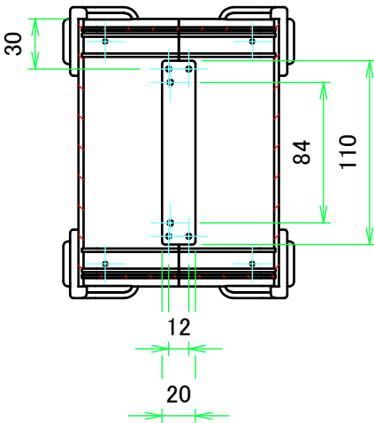
A-A ( 1 : 4 )
