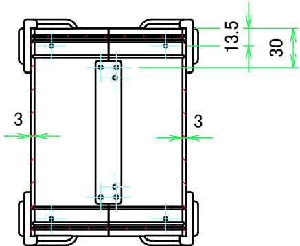
B-B ( 1 : 4 )
