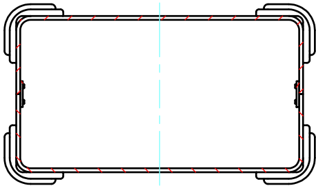
C-C ( 1 : 4 )
