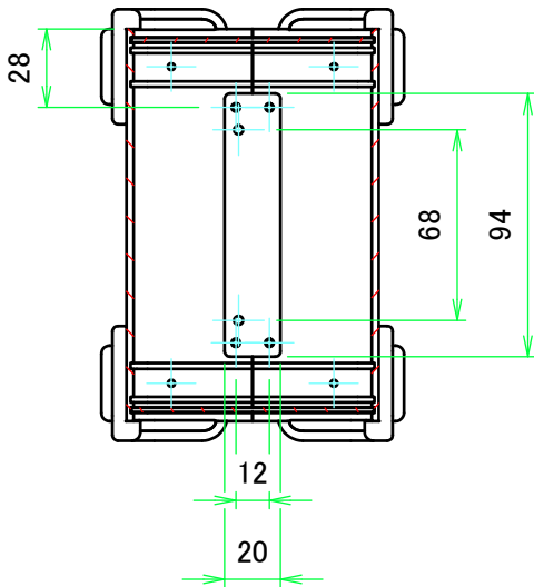
A-A ( 1 : 3 )
