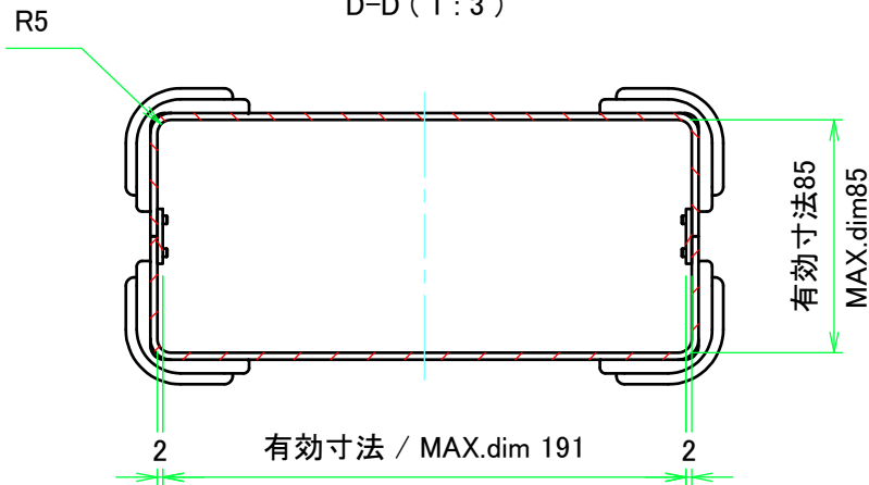
D-D ( 1 : 3 )
