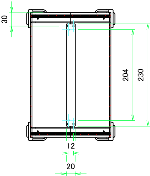
A-A ( 1 : 5 )
