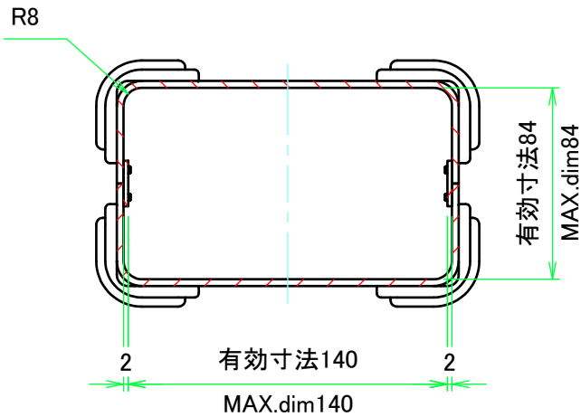
D-D ( 1 : 3 )
