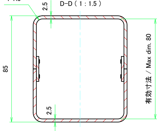
4-R5 D-D ( 1 : 1.5 )
