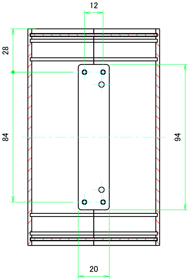
A-A ( 1 : 1.5 )
