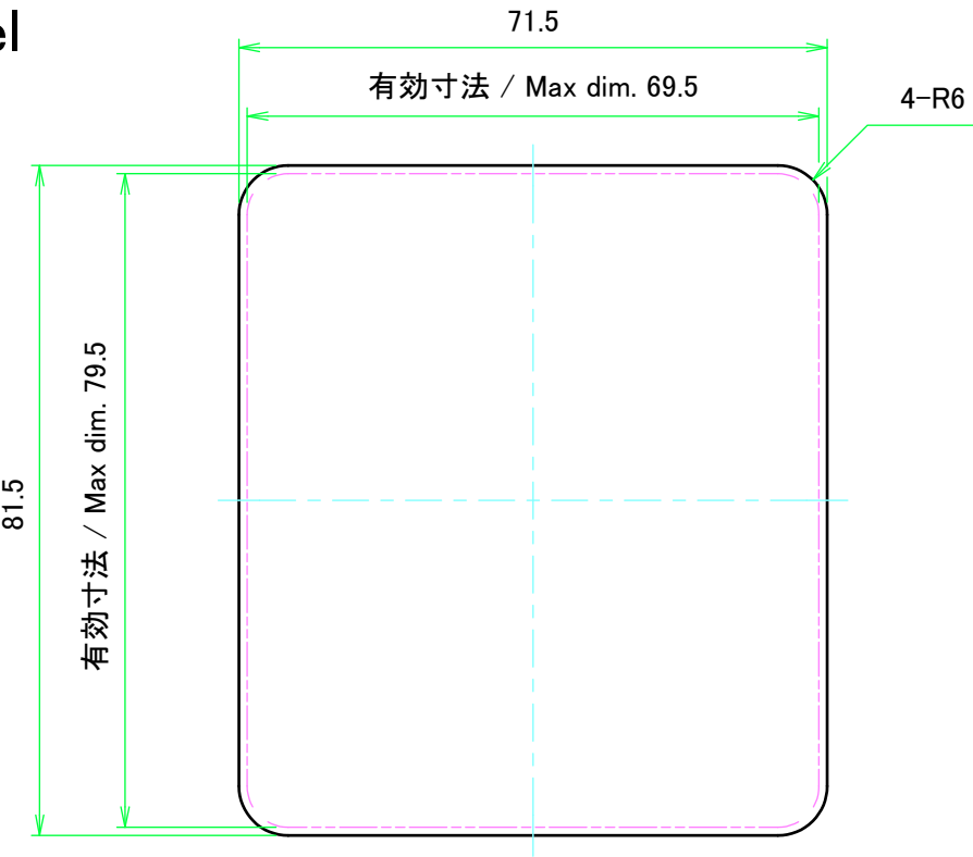
パネル表面 / Panel Frontside
