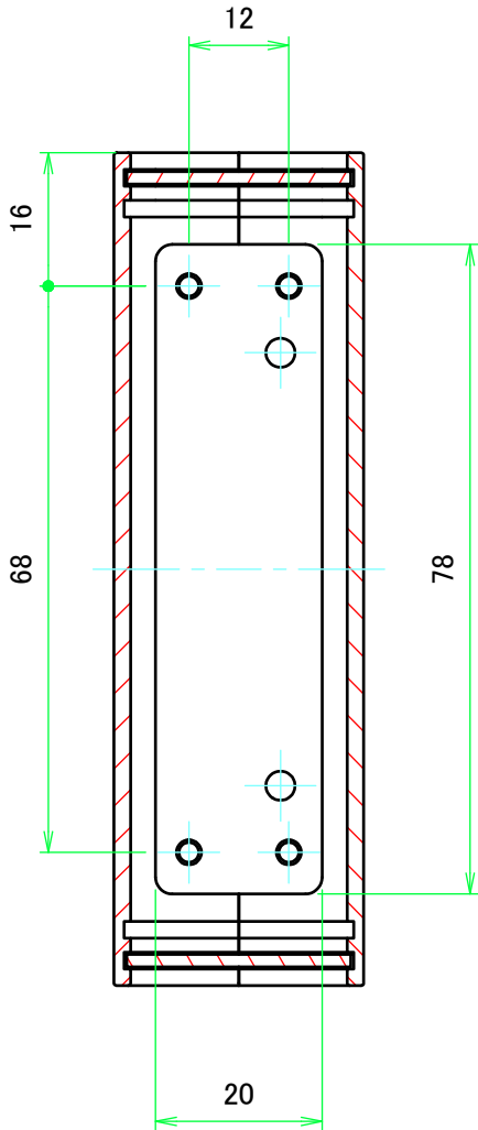
A-A (1:1)
