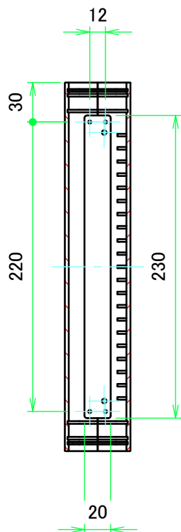
A-A ( 1 : 4 )
