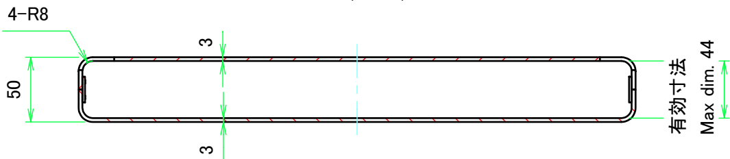
D-D ( 1 : 4 )
