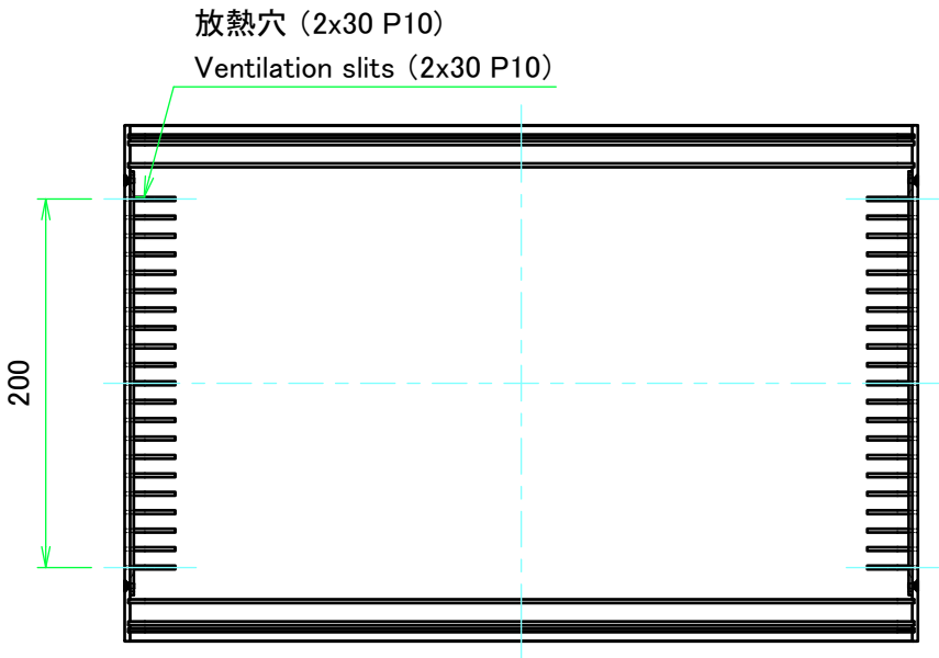
上カバー(内視) Top cover (Internal view)
