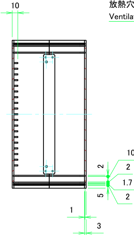
B-B ( 1 : 4 )
