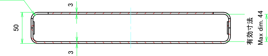
D-D ( 1 : 3 )
