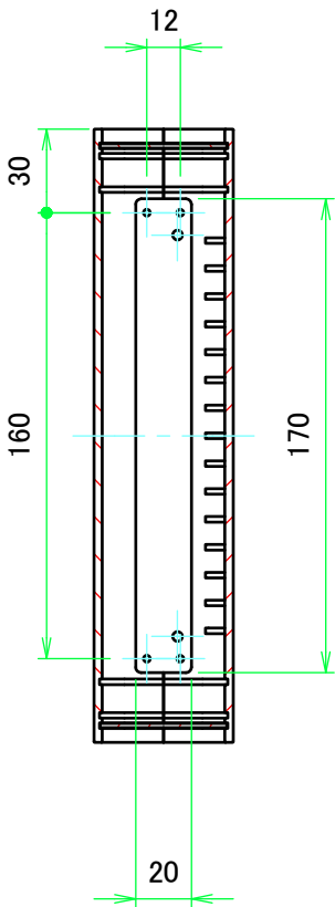
A-A ( 1 : 3 )
