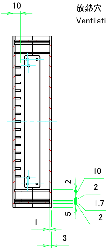
B-B ( 1 : 3 )
