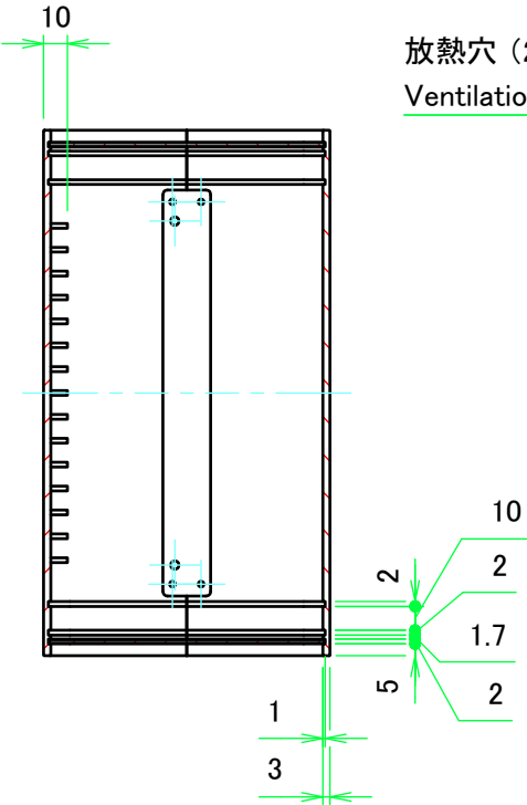
B-B ( 1 : 3.5 )
