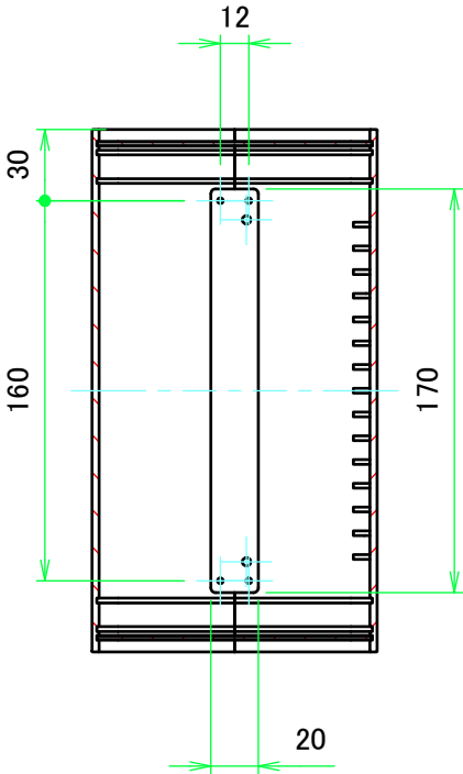
A-A ( 1 : 3.5 )
