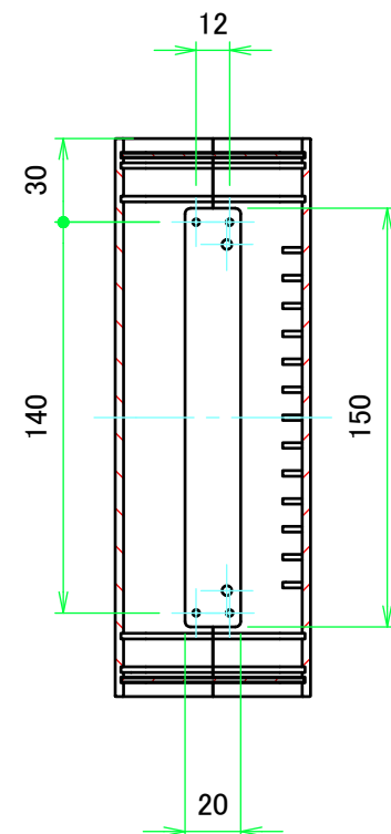
A-A ( 1 : 3 )
