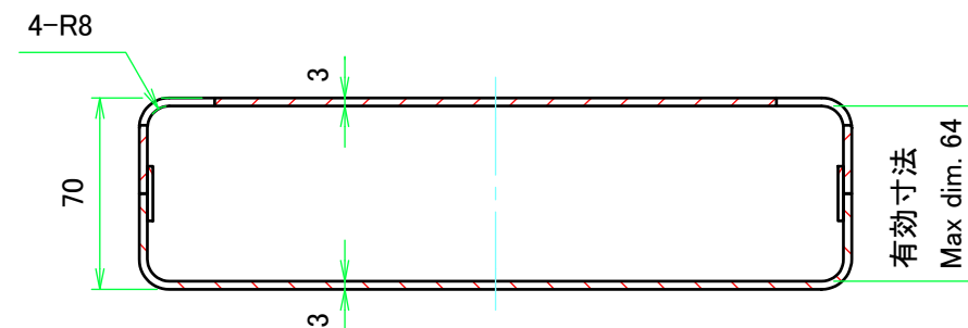
D-D ( 1 : 3 )
