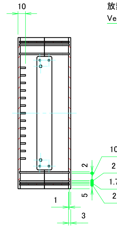
B-B ( 1 : 3 )
