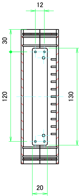
A-A ( 1 : 2.5 )
