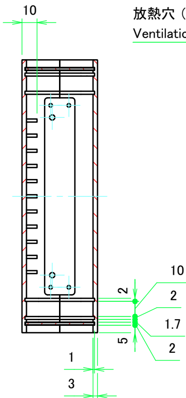
B-B ( 1 : 2.5 )
