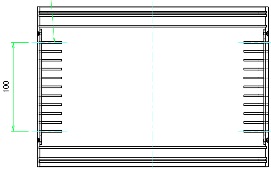
放熱穴 (2x30 P10) Ventilation slits (2x30 P10)
