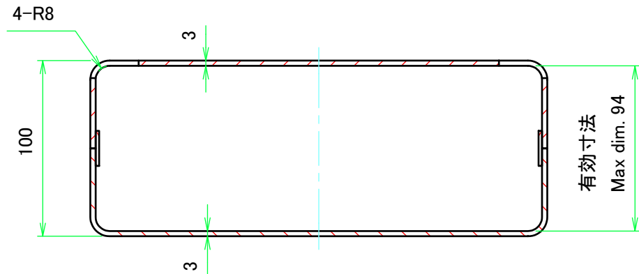
D-D ( 1 : 3 )
