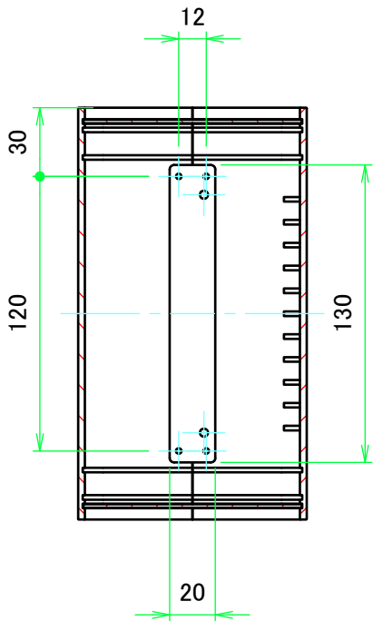
A-A ( 1 : 3 )
