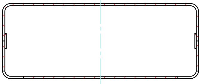
C-C ( 1 : 3 )
