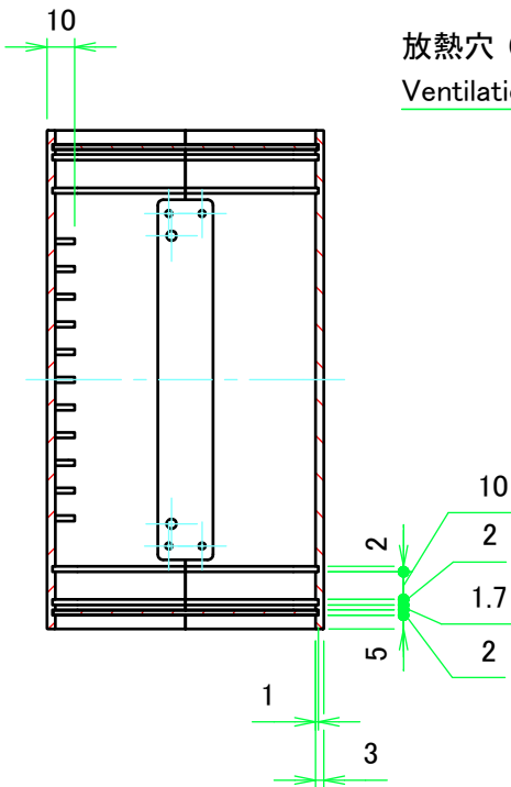
B-B ( 1 : 3 )
