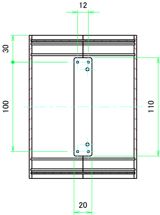
A-A ( 1 : 2.5 )
