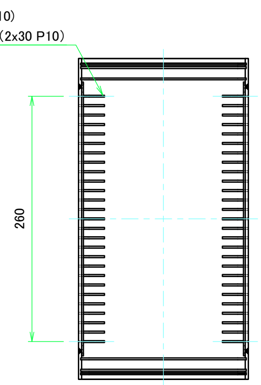
上カバー(内視) Top cover (Internal view)
