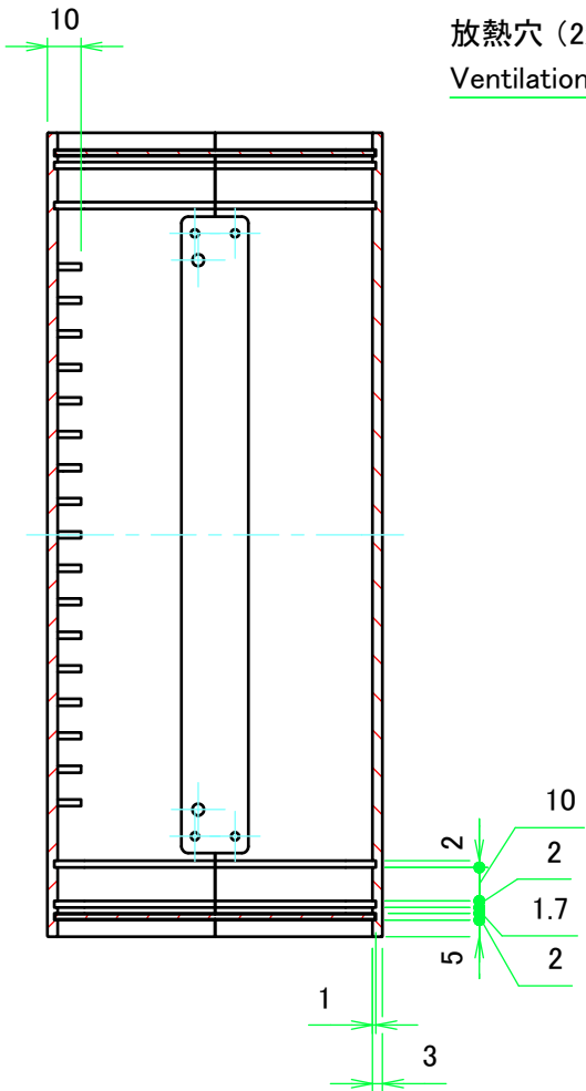
B-B ( 1 : 2.5 )
