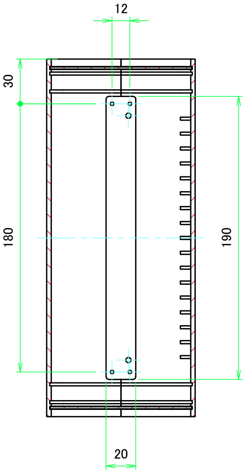
A-A ( 1 : 2.5 )
