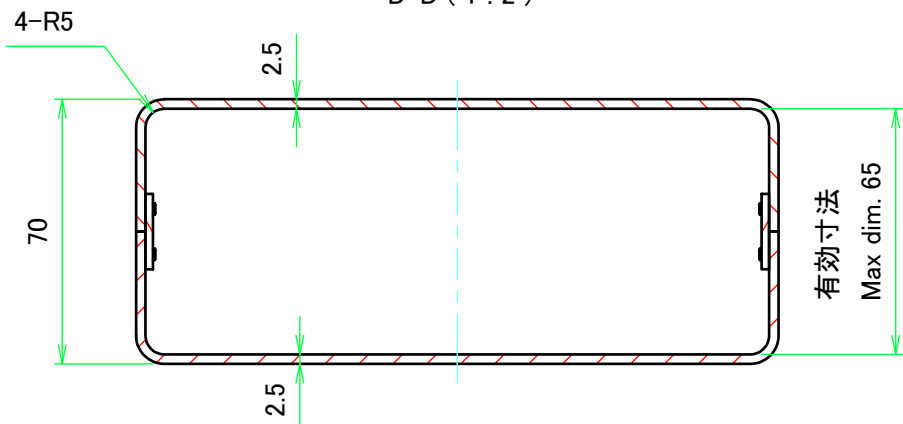
D-D ( 1 : 2 )
