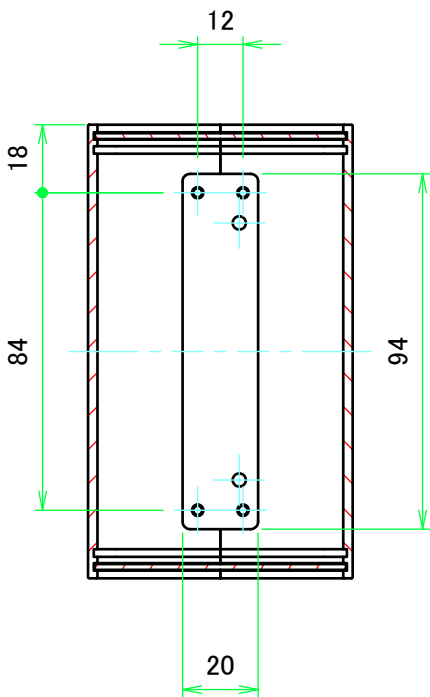
A-A ( 1 : 2 )
