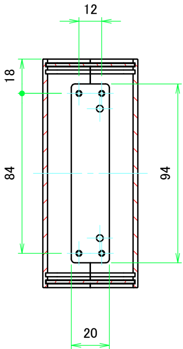
A-A ( 1 : 2 )
