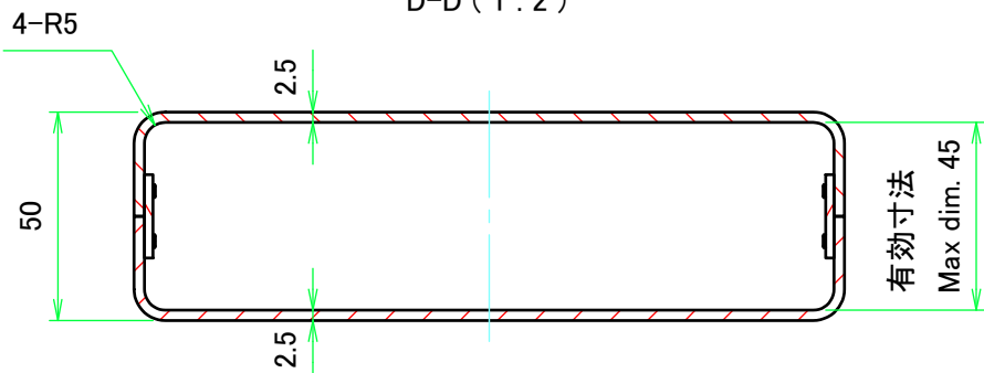
D-D ( 1 : 2 )
