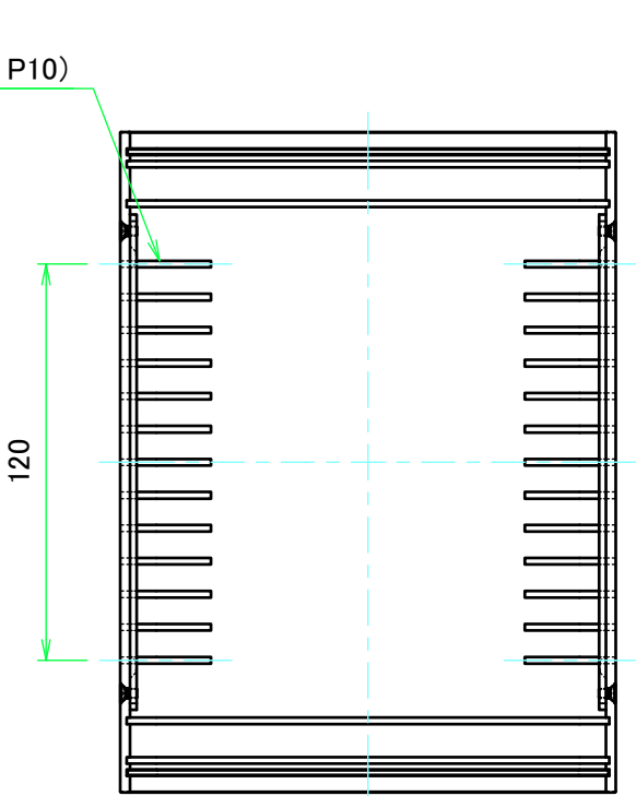
上カバー (内視) Top cover (Internal view)
