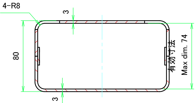
D-D ( 1 : 2.5 )
