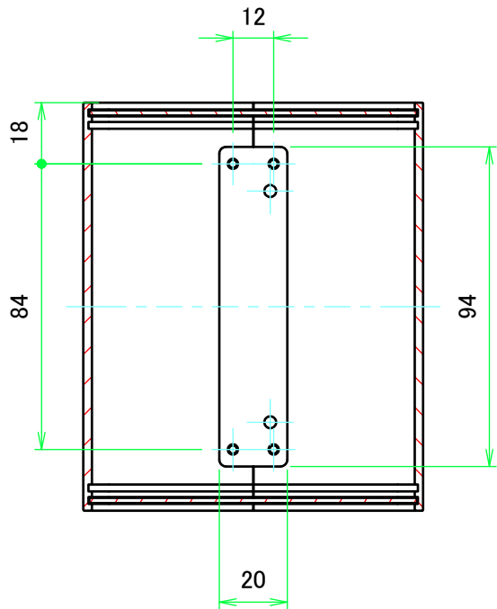
A-A ( 1 : 2 )
