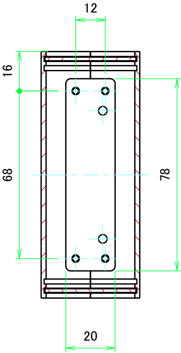
A-A ( 1 : 1.5 )
