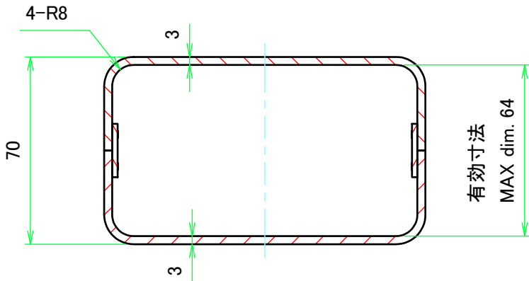
D-D ( 1 : 2 )
