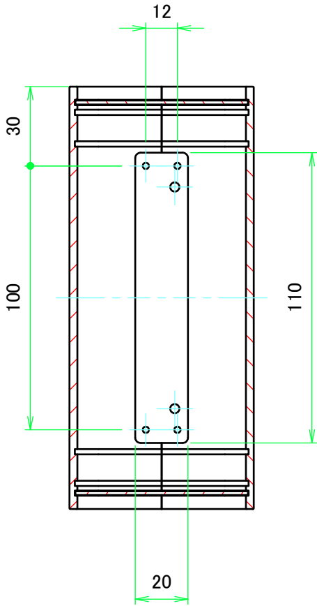
A-A ( 1 : 2 )
