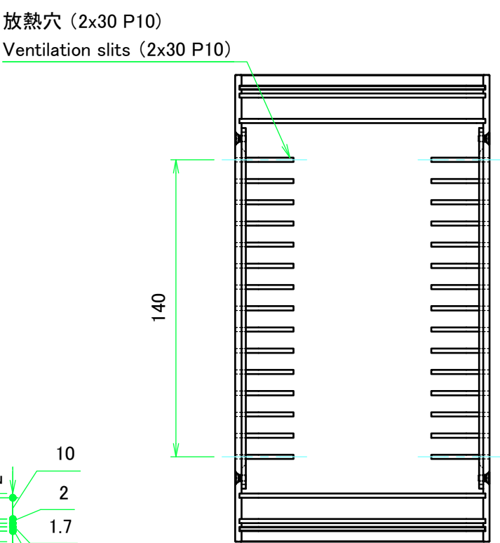
上カバー(内視) / Top cover (Internal view)
