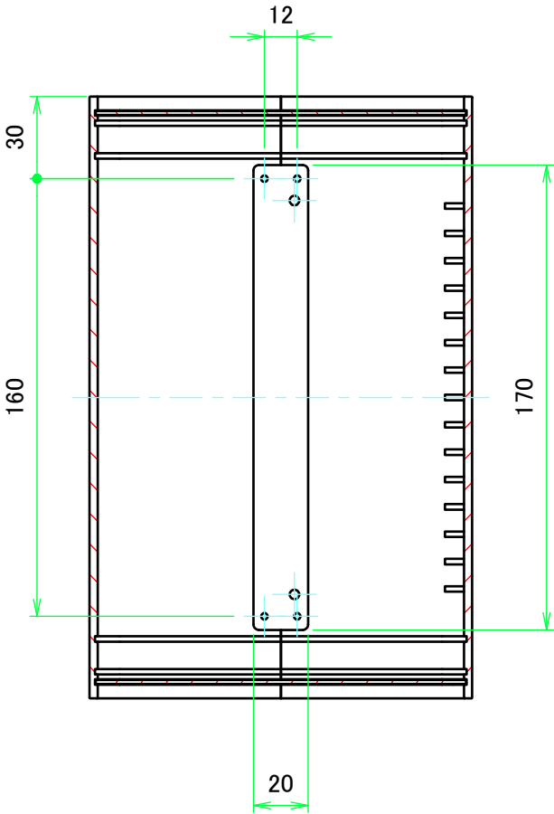
A-A ( 1 : 2.5 )
