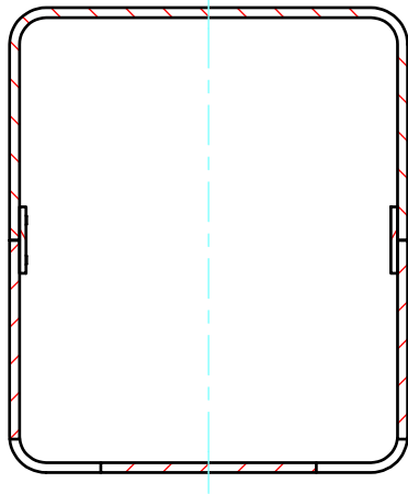
C-C ( 1 : 2.5 )
