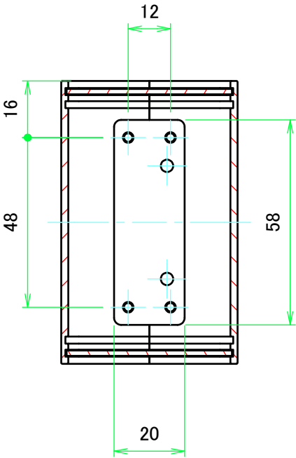
A-A ( 1 : 1.5 )
