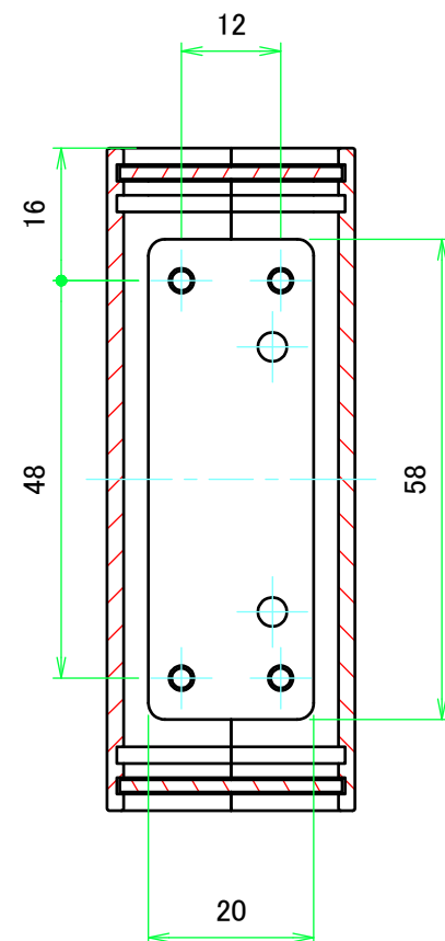
A-A ( 1 : 1 )
