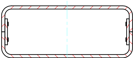
C-C ( 1 : 1.5 )
