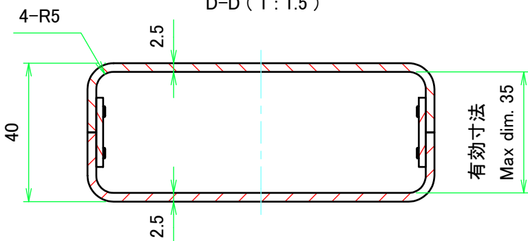
D-D ( 1 : 1.5 )
