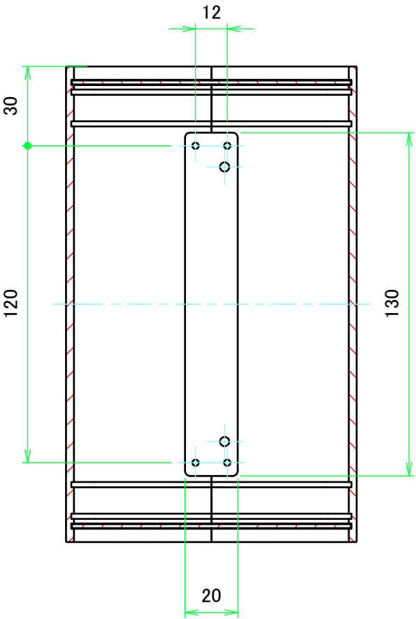
A-A ( 1 : 2 )
