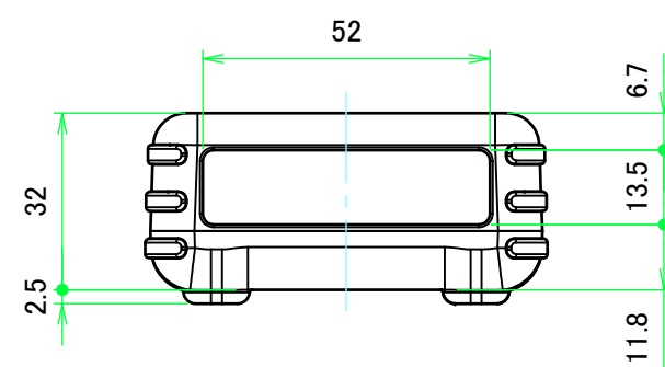
B-B ( 1 : 1.5 )
