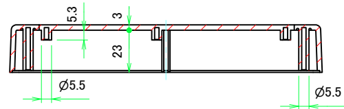
D-D (1:2)
