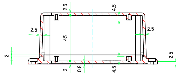
B-B (1 : 1.5)
