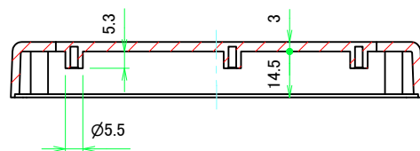
D-D (1:1.5)
