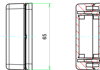
A-A (1 : 1.5)
