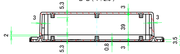
B-B (1:2.5)
