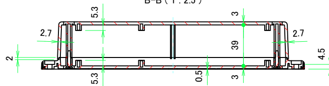
B-B (1:2.5)
