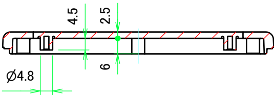
D-D ( 1 : 1.5 )
