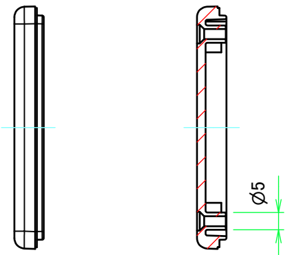
C-C ( 1 : 1.5 )
