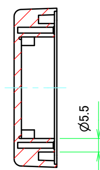
E-E ( 1 : 1.5 )
