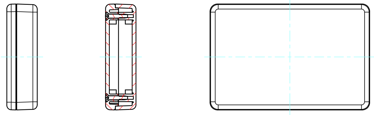
A-A ( 1 : 1.5 )
