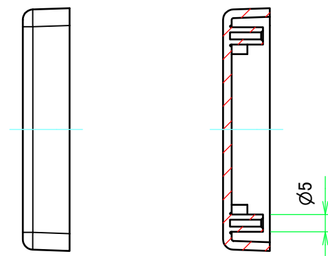
E-E ( 1 : 1.5 )
