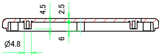
D-D ( 1 : 1.5 )
