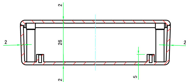
B-B ( 1 : 1.5 )
