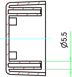
D-D ( 1 : 1.5 )
