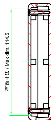
A-A ( 1 : 2.5 )
