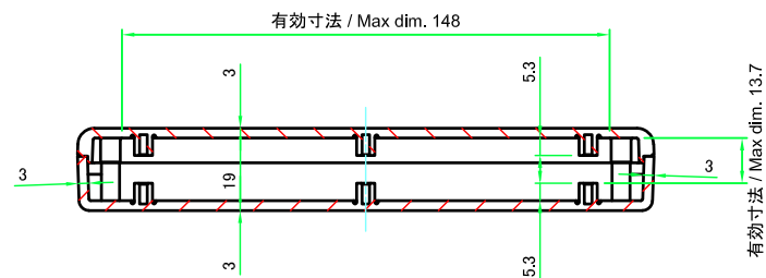
B-B ( 1 : 2.5 )
