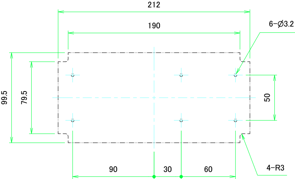
推奨基板形状 * 販売していません Recommended PCB dimension * NOT SUPPLIED
